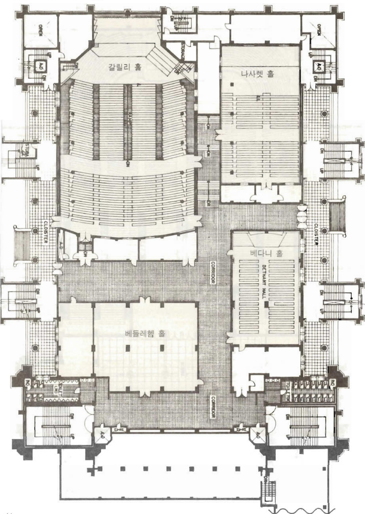
본당 1층 평면도
